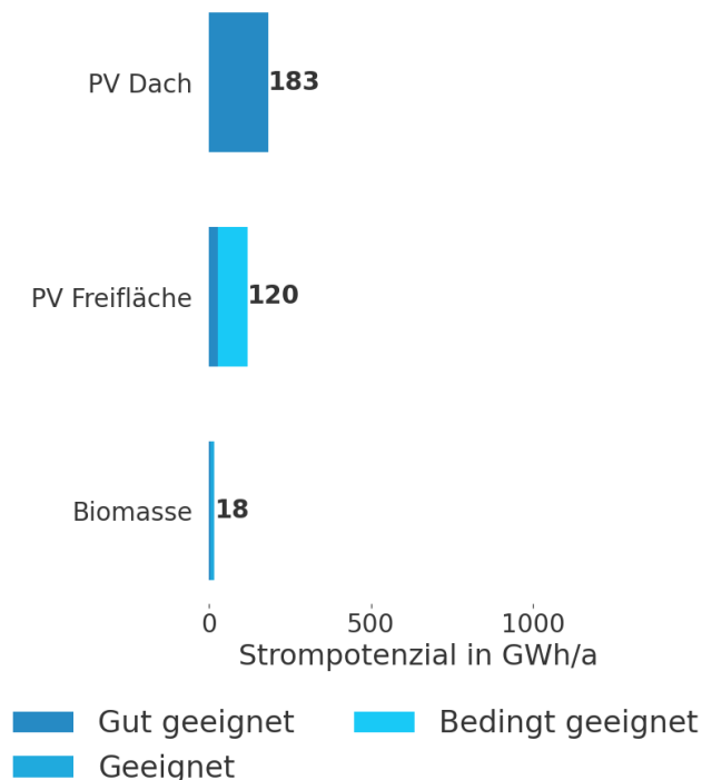
Abbildung 20: Erneuerbare Strompotenziale in Dreieich
