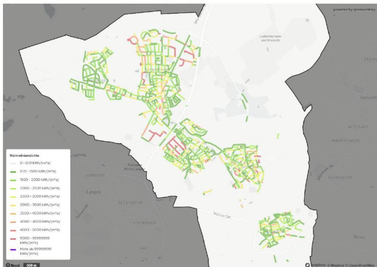
Abbildung 28: Wärmelinienichte im Zieljahr 2040
