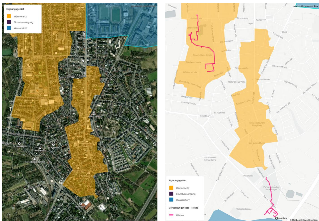
Abbildung 38: Prioritäre Maßnahme 2 – Realisierung eines Wärmenetzes in Sprendlingen Mitte
