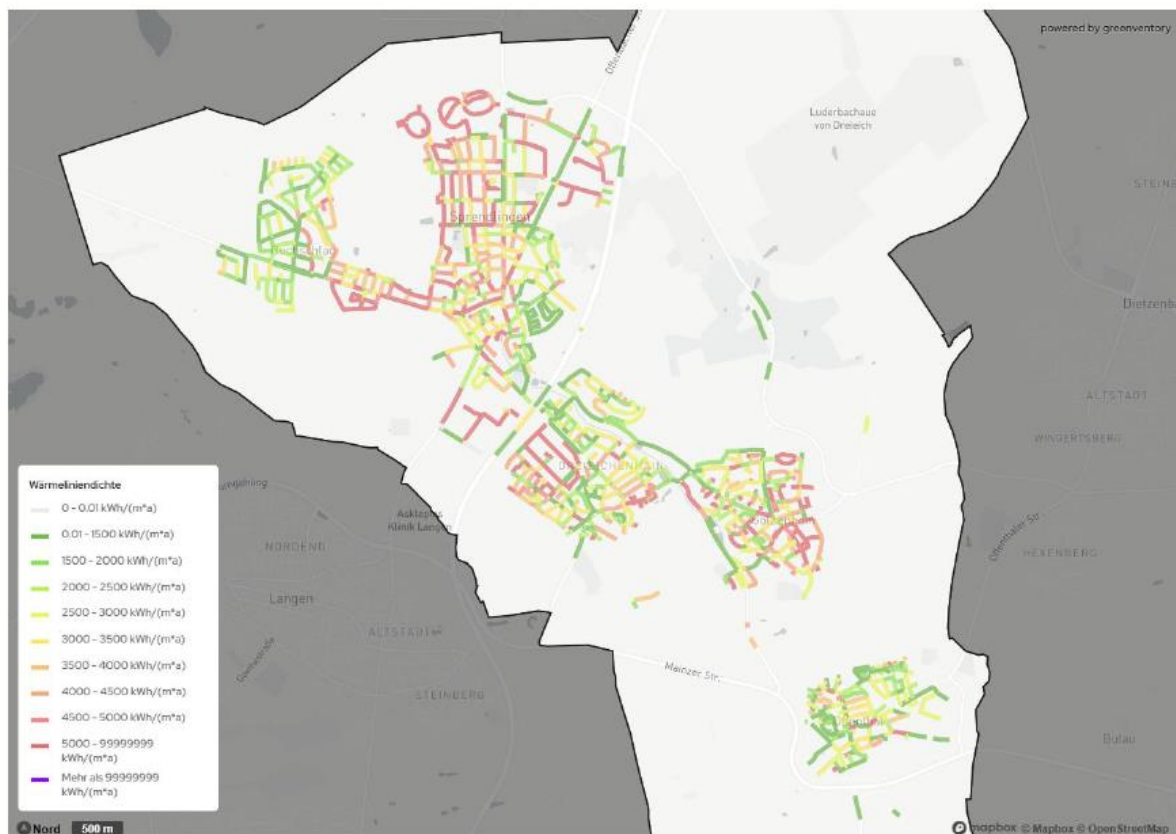
Abbildung 8: Wärmeliniendichte im Status Quo
