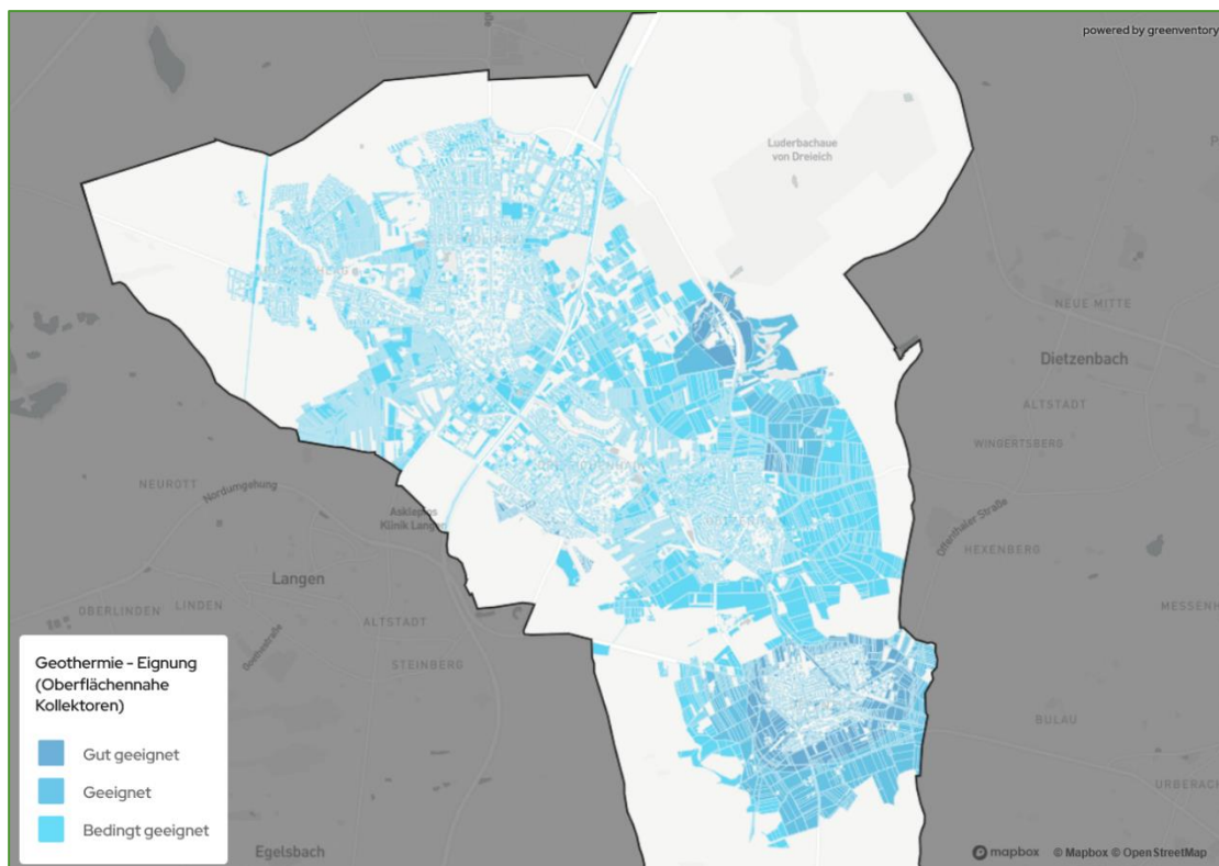
Abbildung 44: Wärmerzeugungspotenzial der oberflächennahen Geothermie (Erdwärmekollektoren) in Dreieich
