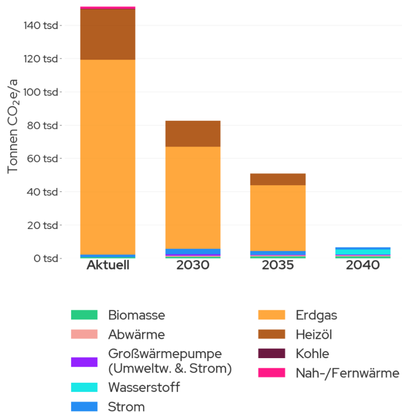
Abbildung 35: Entwicklung der Treibhausgasemissionen
