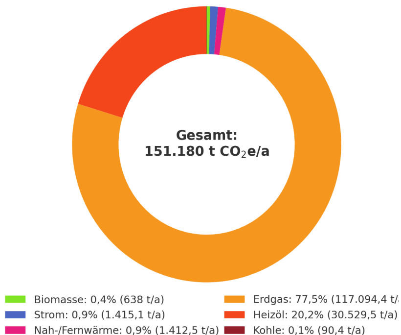
Abbildung 16: Treibhausgasemissionen nach Energieträger im Projektgebiet
