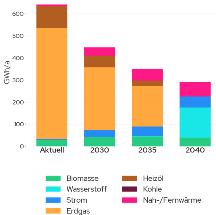
Abbildung 27: Reduktionspotenzial des Endenergiebedarfs für die Stadt Dreieich im Zieljahr 2040
