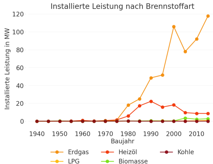
Abbildung 9: Gesamtleistung der jährlich neu installierten Heizsysteme im Bestand nach Energieträger, gruppiert in 5-Jahresabschnitten (Summe)
