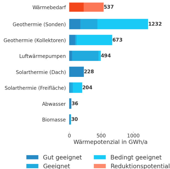
Abbildung 21: Erneuerbare Wärmepotenziale in Dreieich
