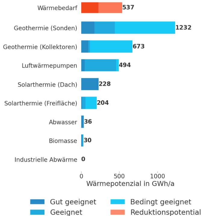
Abbildung 24: Übersicht der Potenziale zur Wärmeerzeugung in der Stadt Dreieich
