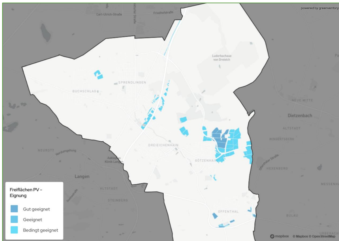
Abbildung 42: Stromerzeugungspotenzial der Freiflächen-PV in Dreieich
