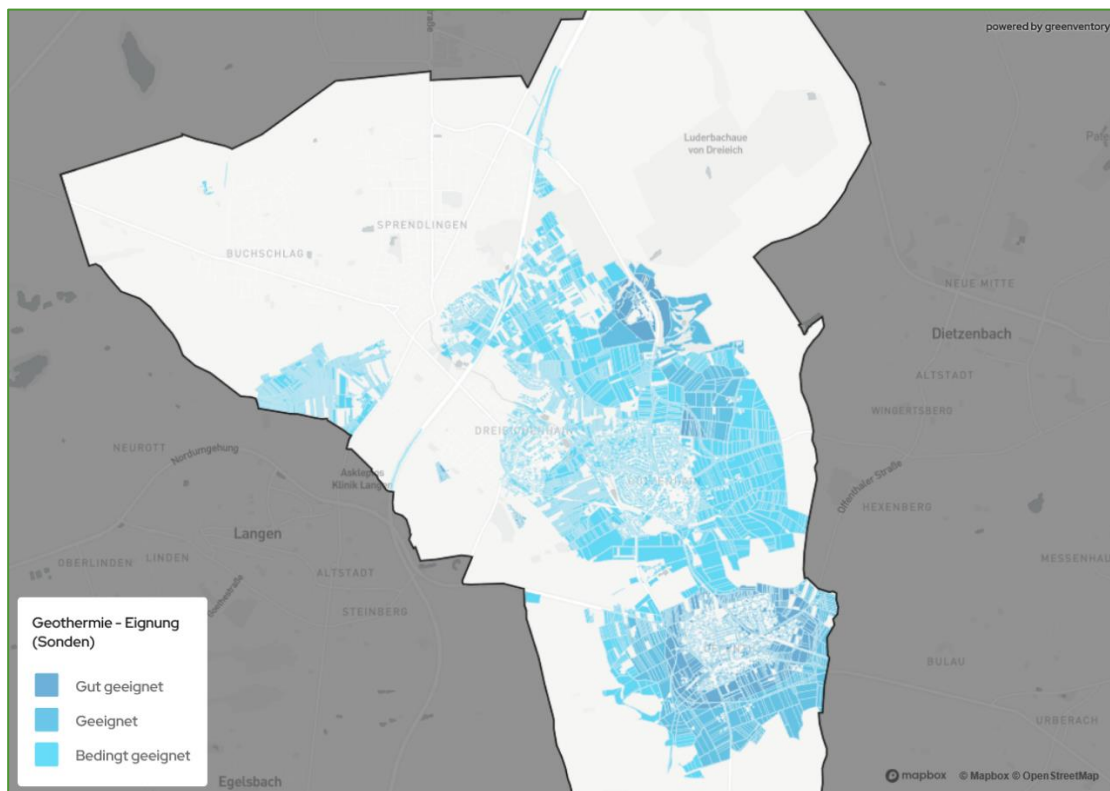
Abbildung 43: Wärmerzeugungspotenzial der oberflächennahen Geothermie (Erdwärmesonden) in Dreieich
