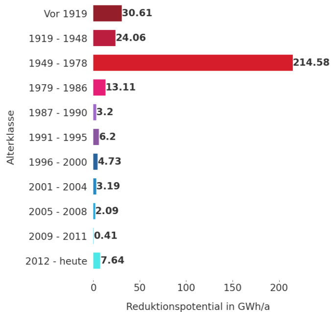
Abbildung 22: Reduktionspotenzial nach Baualtersklassen
