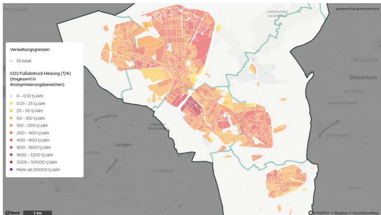
Abbildung 17: Verteilung der Treibhausgasemissionen in Dreieich
