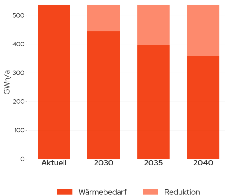
Abbildung 26: Reduktionspotenzial des Wärmebedarfs
