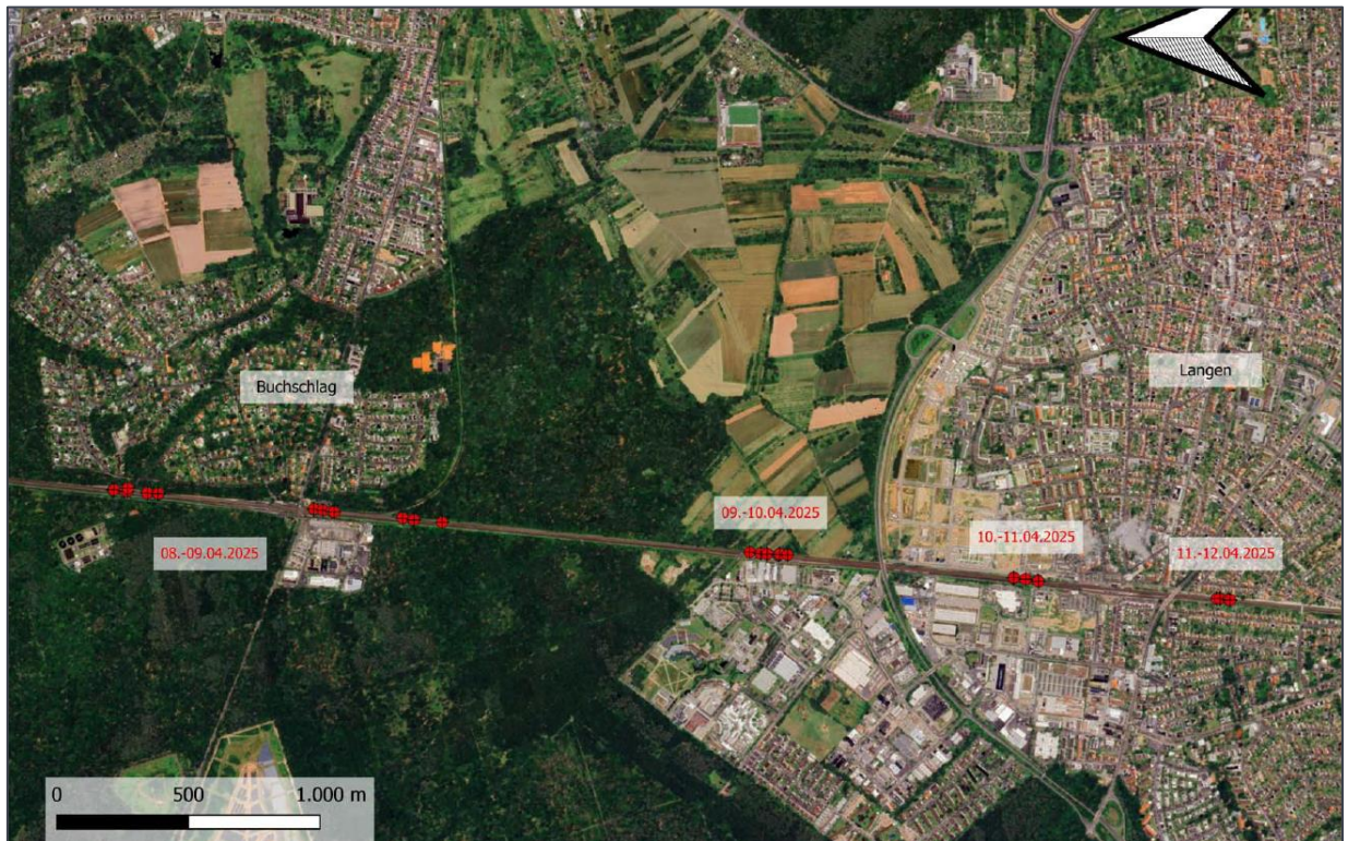
Bohrpunkte der Baugrunderkundungen auf der Main-Neckar-Bahn vom 8. - 12. April 2025
